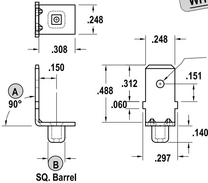
OPTION 2 + 5 90°
